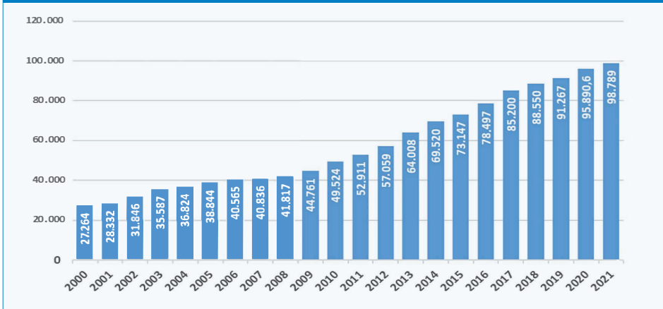
GRAFİK 2. TÜRKİYE'DE ELEKTRİK ENERJİSİ KURULU GÜÇ GELİŞİMİ (2000-2021*, MEGAWATT/MW)**
