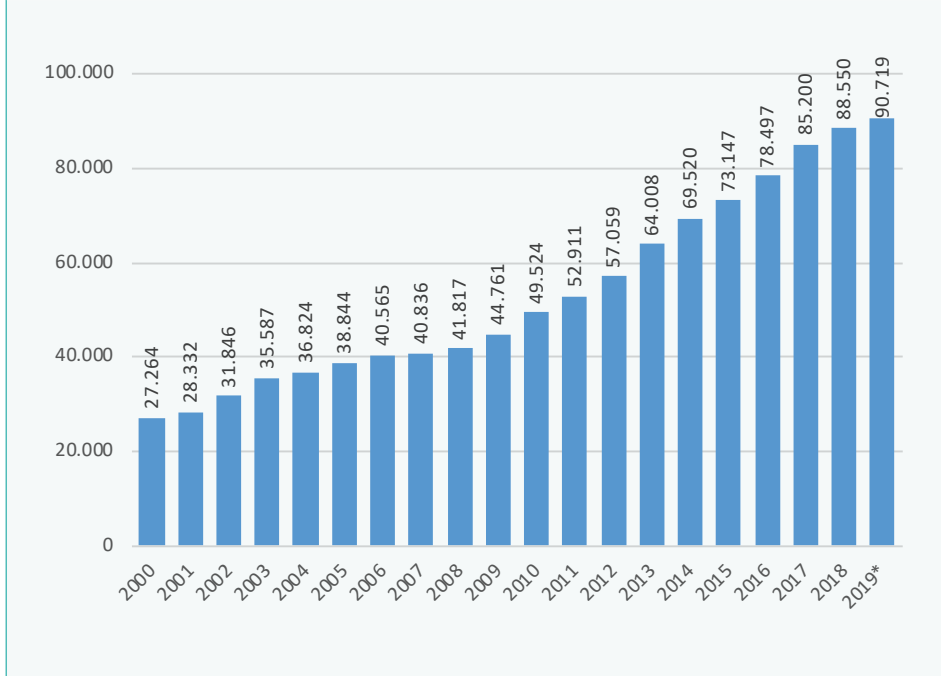
GRAFİK 2. TÜRKİYE'NİN ELEKTRİK ENERJİSİ KURULU GÜÇ GELİŞİMİ (2000-2019, MW)
